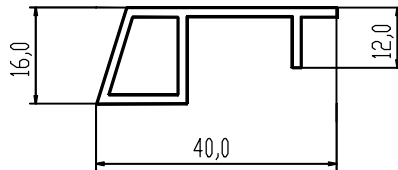
KAP 4016-S
