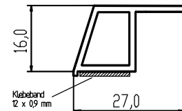
KA 2716-S
