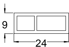
KA 2409
