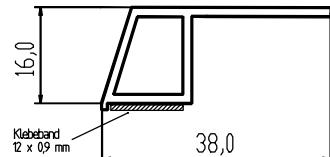
KA 3816-S
