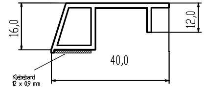
KAP 4016-S
