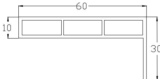
KA 601030
