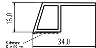
KA 3416-S
