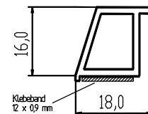
KA 1816-S
