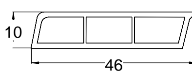
KA 4610
