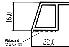
KA 2216-S
