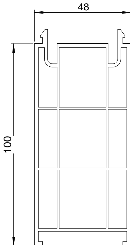
UB 48100 Unterbauprofil
