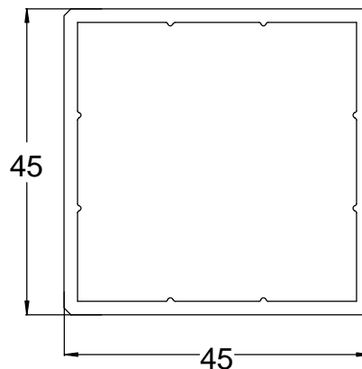
R 4545 Wandstärke 2,0 mm
