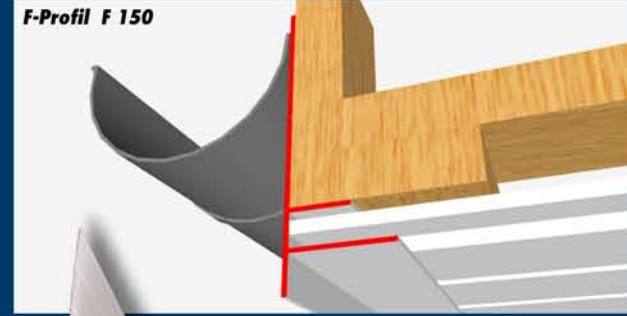
F-Profil F 150
